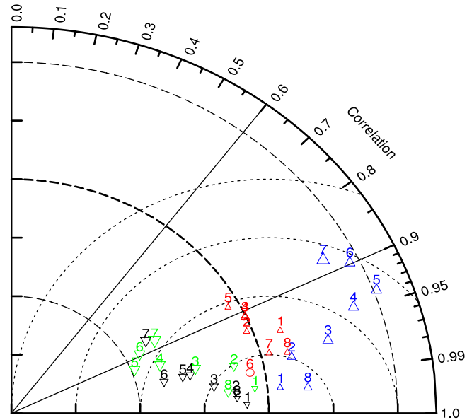
(d) Shortwave radiation
