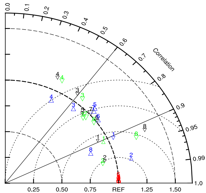
(d) Shortwave radiation
