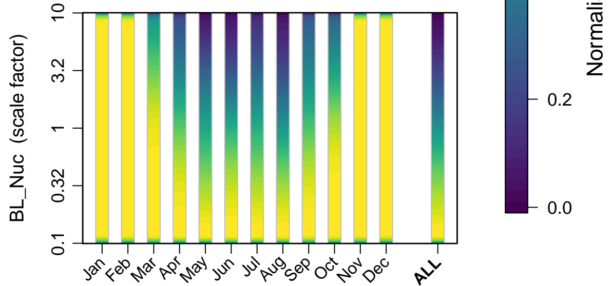
(d) BL_Nuc constrained by N 3
