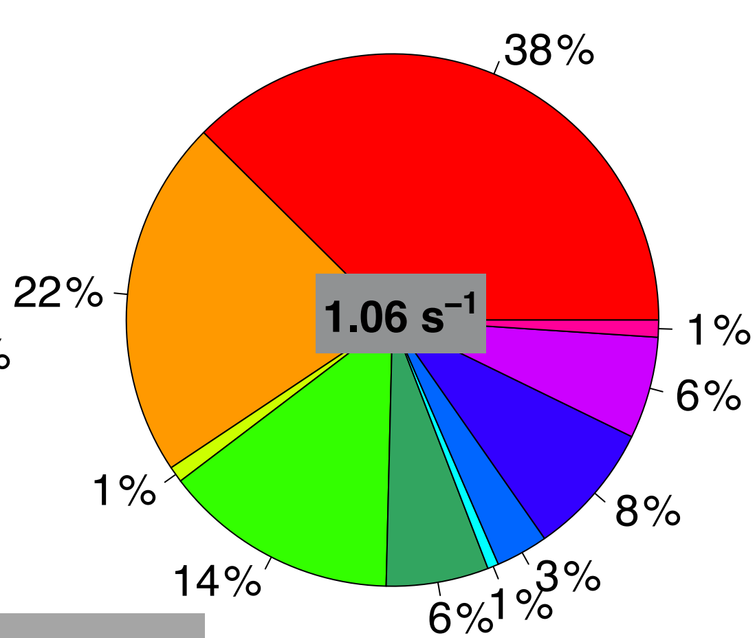
Model (NH)
