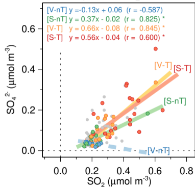
(a) \text{SO}_4^{2-} vs. \text{SO}_2
