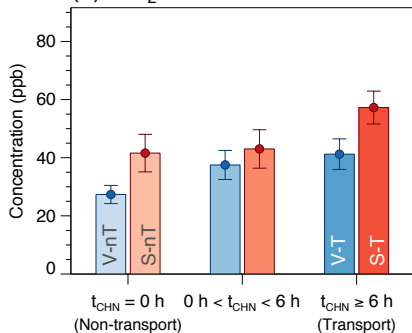
(b) NO 2
