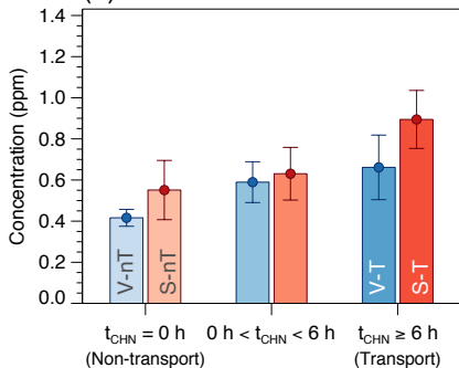
(d) CO
