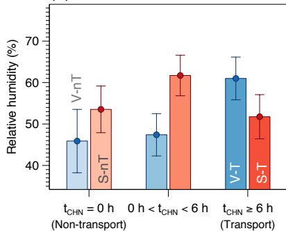
(b) RH
