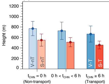
(d) BLH
