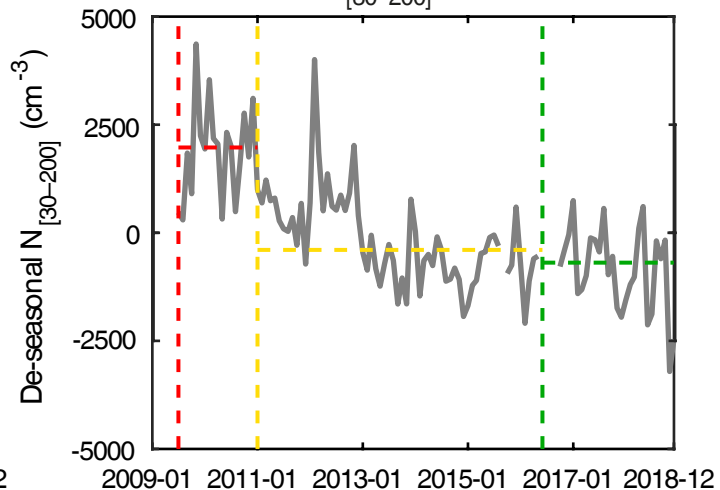
(d) N_{[30-200]} at LTR
