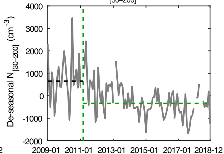
(d) N_{[30-200]} at LTR
