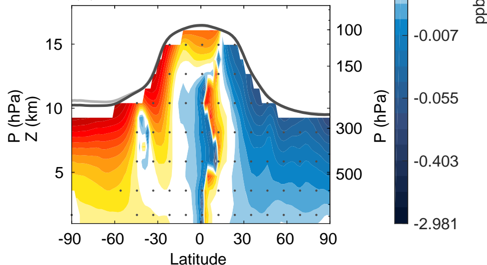
(d) st80 trends WACCM fGHG
