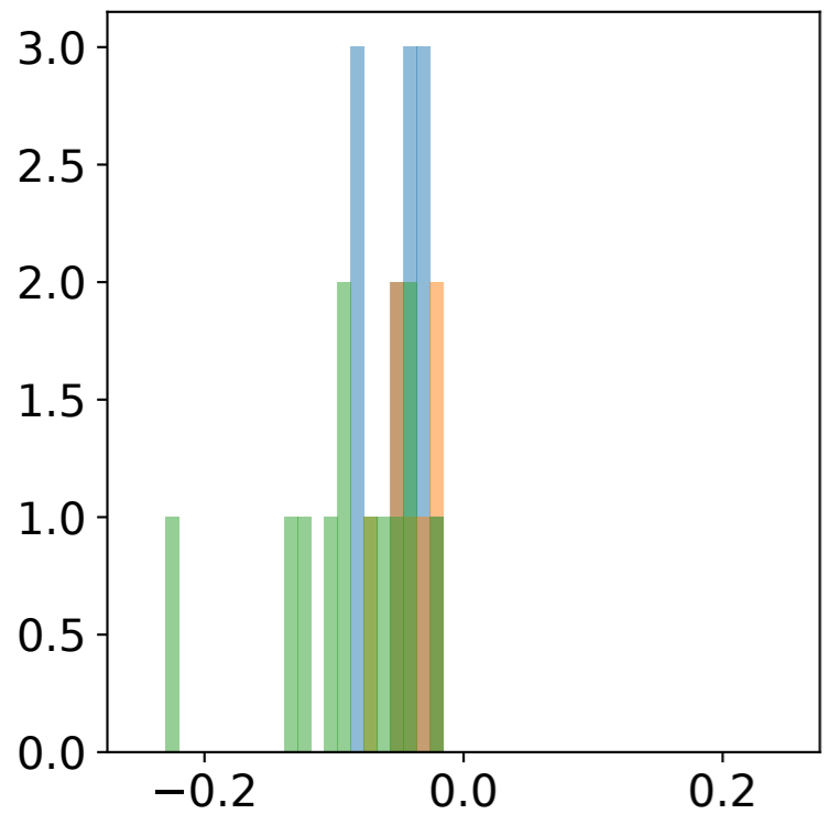
(e) \delta LTS [K]
