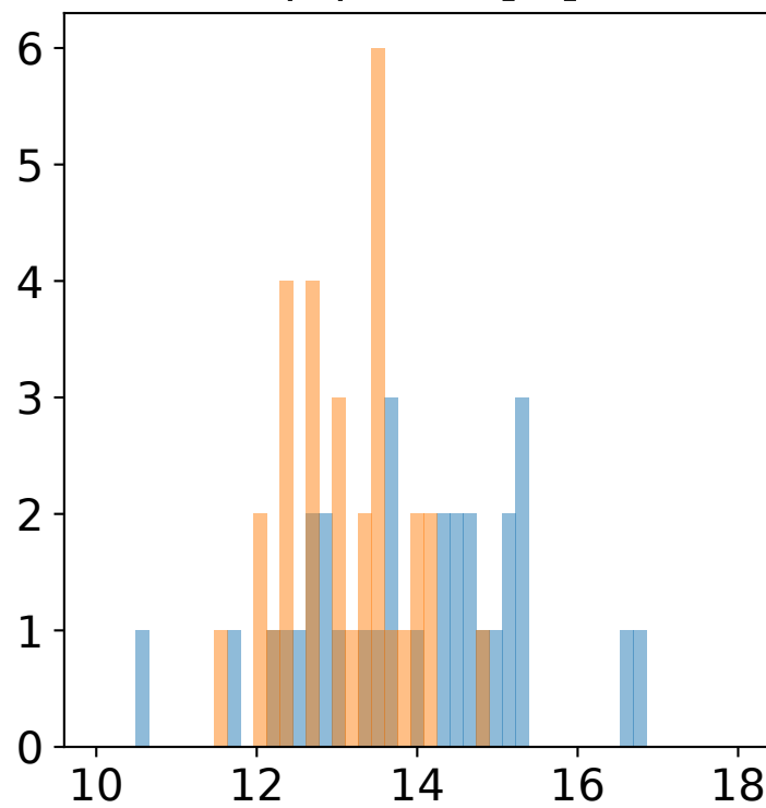
(e) LTS [K]
