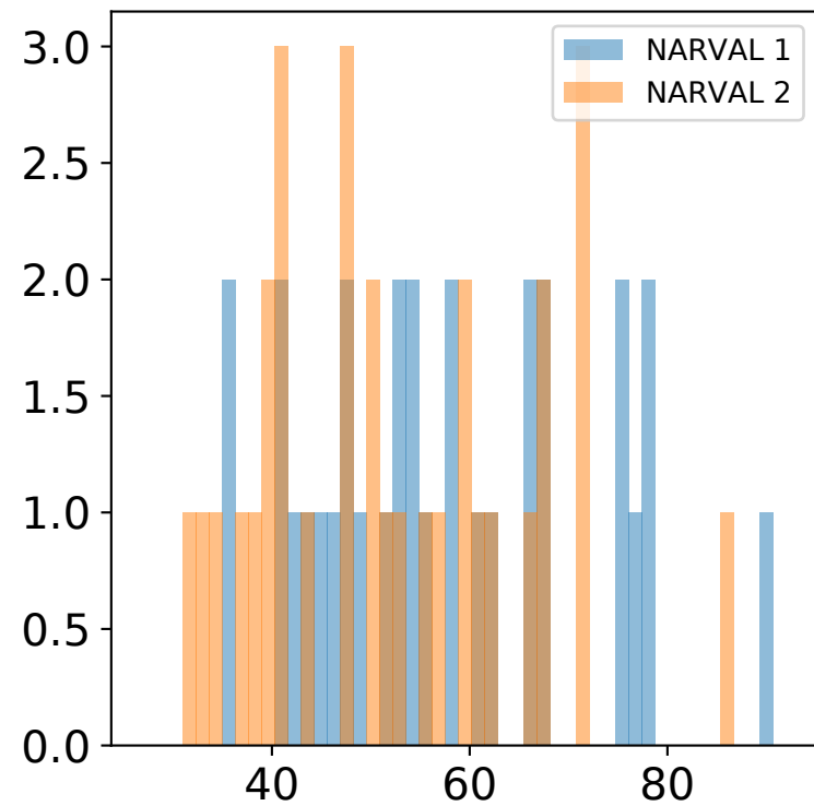
(e) LTS [K]
