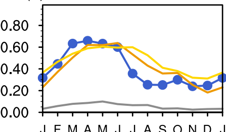
(d) Banizoum 13.5° N, 2.7° E
