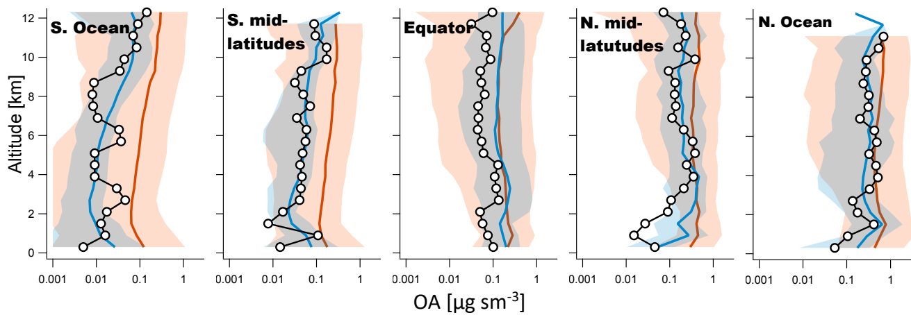
(b) ATom-2
