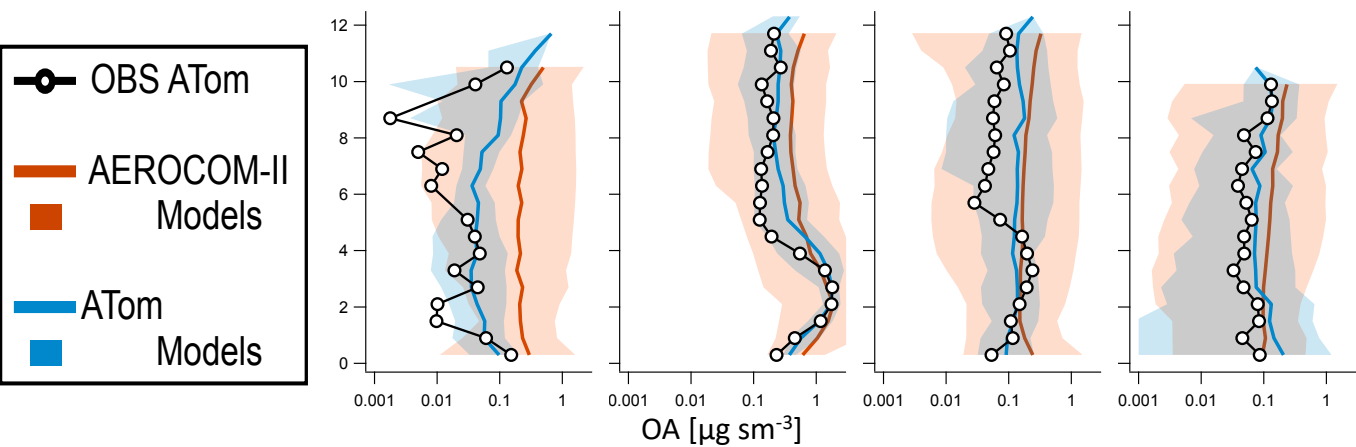
(d) ATom-2
