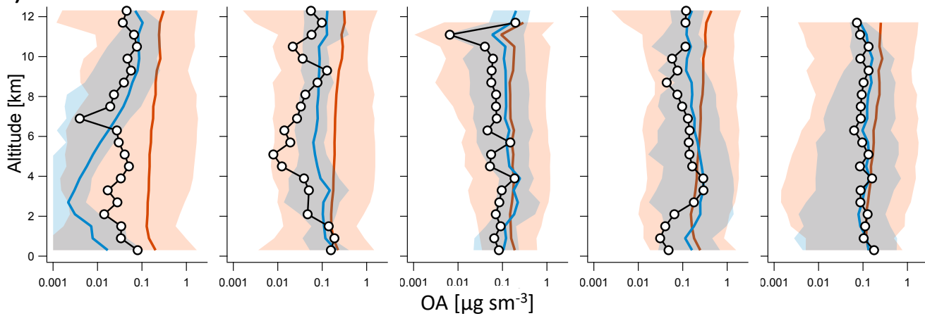
(b) ATom-2
