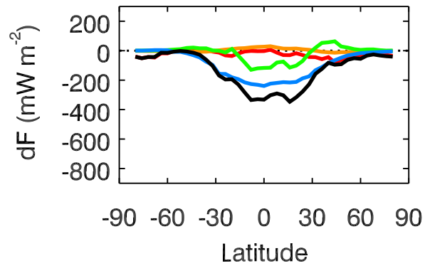
ENS
