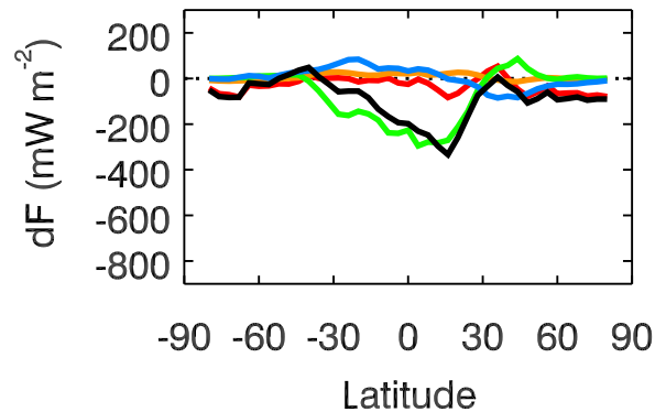
CESM
