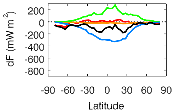
CMAM
