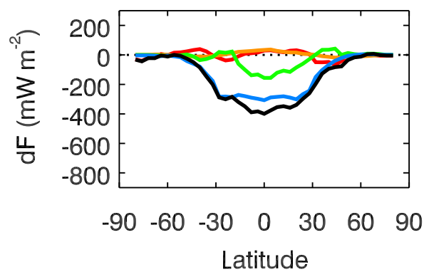
CESM
