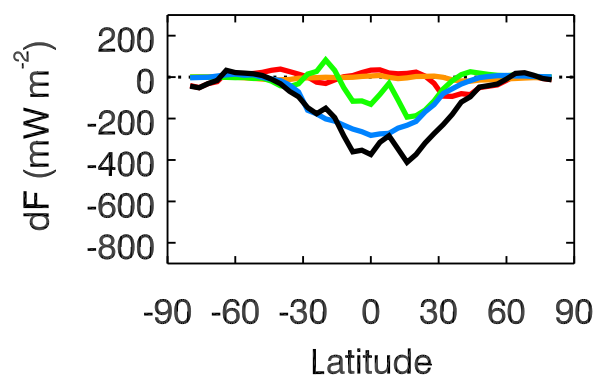
ENS
