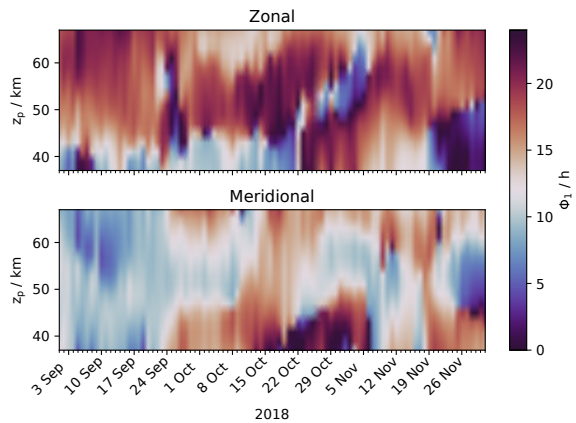
(d) MERRA-2 composite phase \Phi_1
