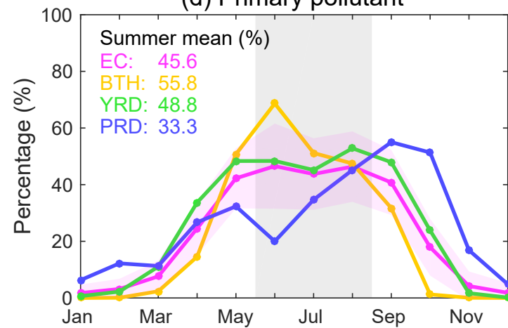
(d) Primary pollutant
