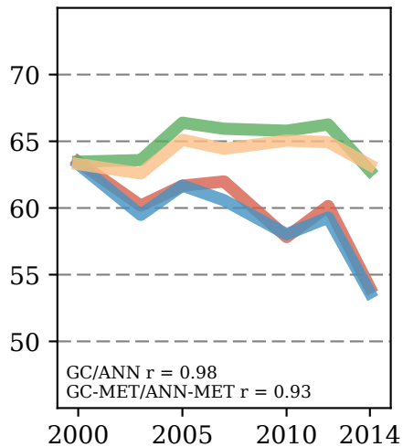
AOT40 wheat MAM [ppmh]
