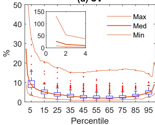
(d) CV
