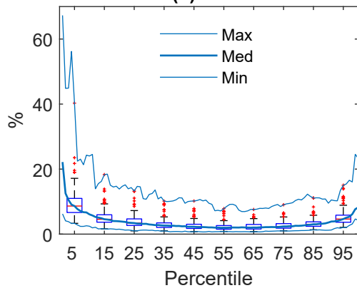
(e) NME
