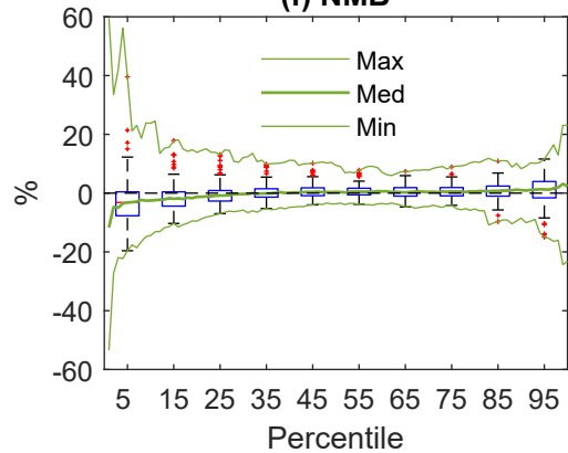
(f) NMB
