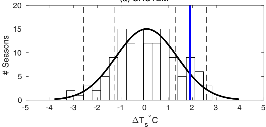
(b) GISTEMP
