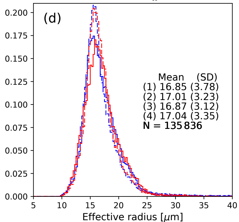
60-120° E JJA
