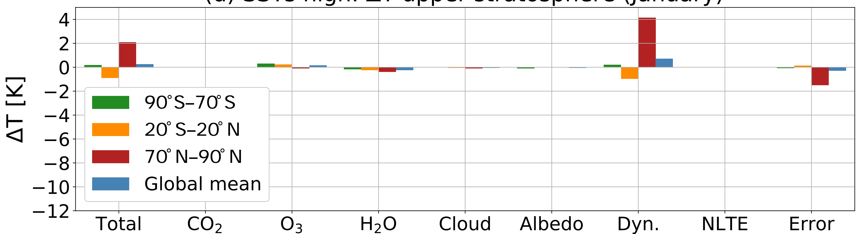
(d) SSTs high: \Delta T upper stratosphere (January)
