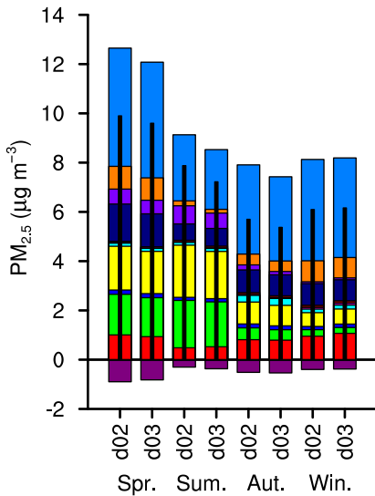
(b2) PM 2.5 (AM)
