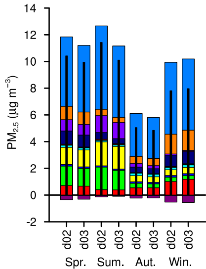
(b1) PM 2.5 (OH)
