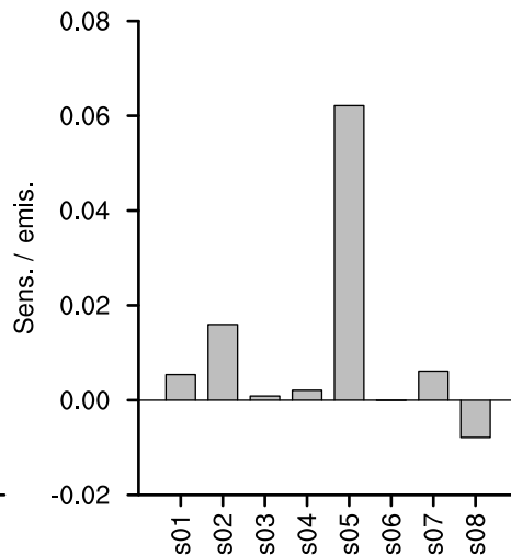
(f) SOA sens. / NMVOC emis.
