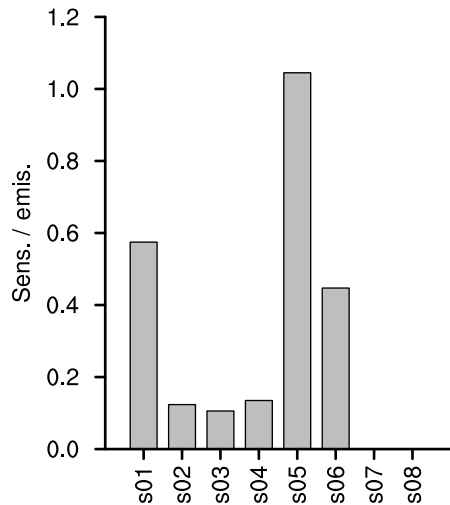
(d) EC sens. / EC emis.
