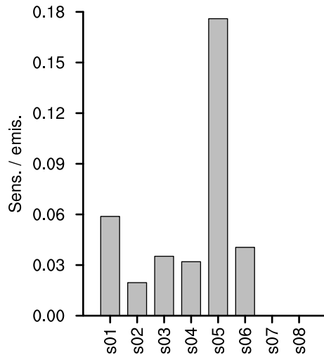
(e) POA sens. / POA emis.
