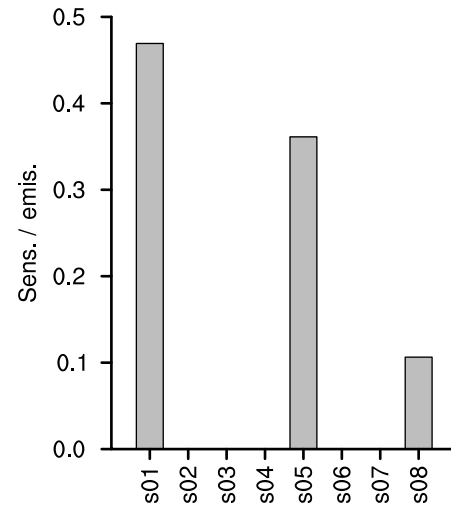
(f) SOA sens. / NMVOC emis.
