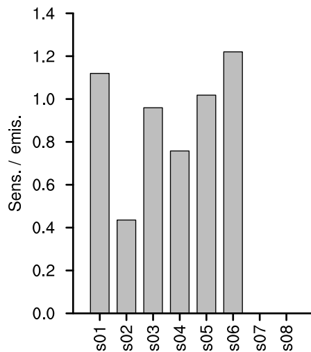
(e) POA sens. / POA emis.
