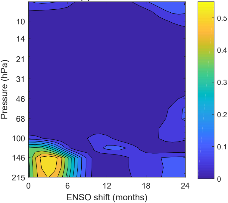
(a) ENSO R^2
