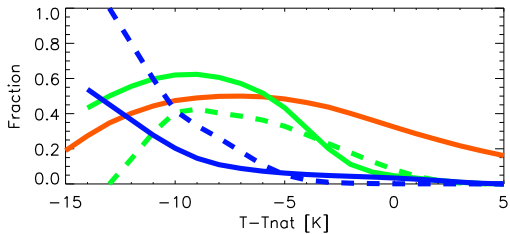
WACCM
