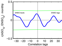
(e) WACCM-R3-2052-2092
