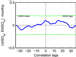
(g) NIWA-R3-2011-2051
