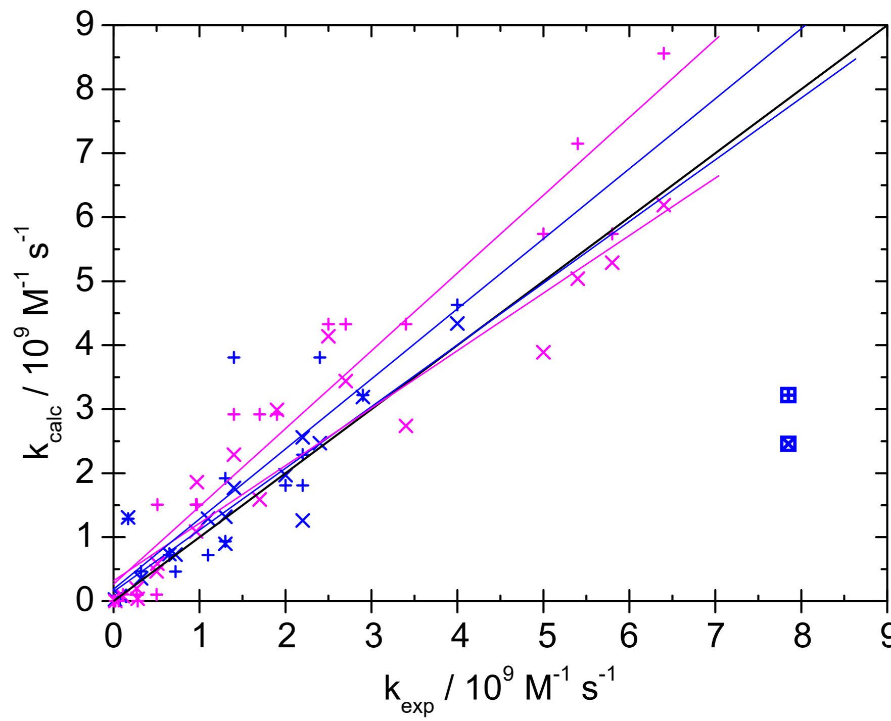
(d) Carboxylic acids
