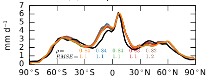
(d) Precipitation
