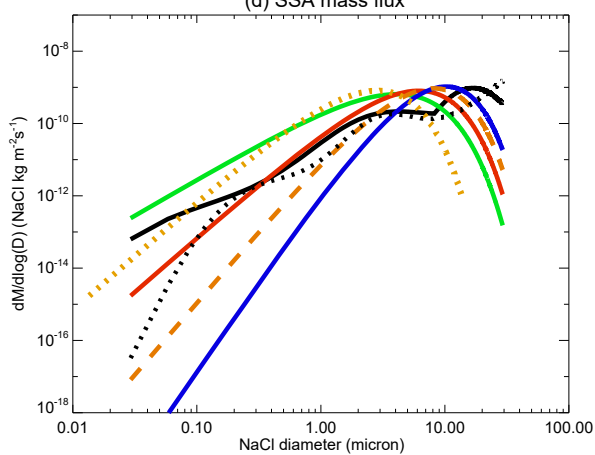
(d) SSA mass flux
