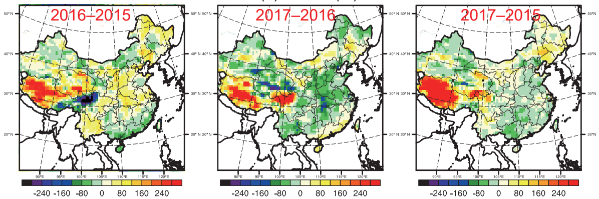
(b) PSFC (Pa)
