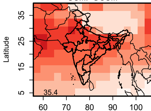
CCMI-GCCM
