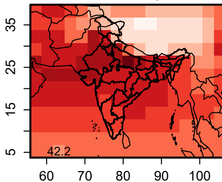
HTAPII-HDGM
