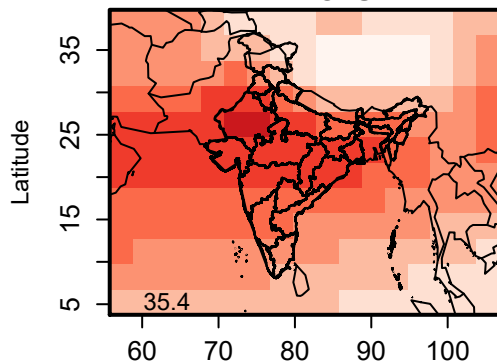
HTAPII-CHSR
