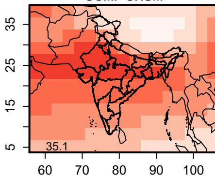
CCMI-CHSM
