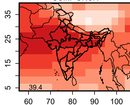
CCMI-UKCA
