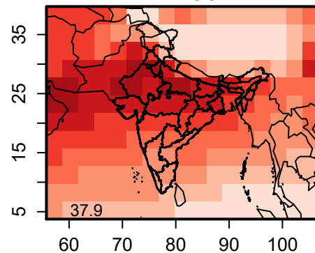
HTAPII-GCAD
