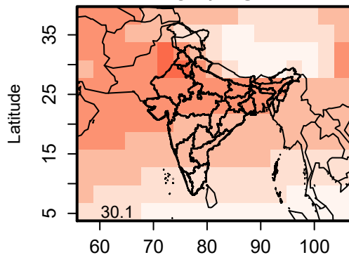
OMI/MLS
