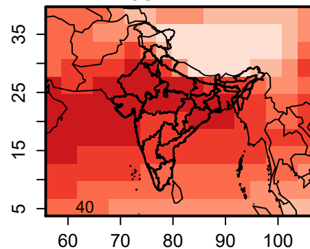
CCMI-MRIE
