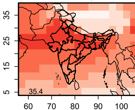
HTAPII-MOZT
