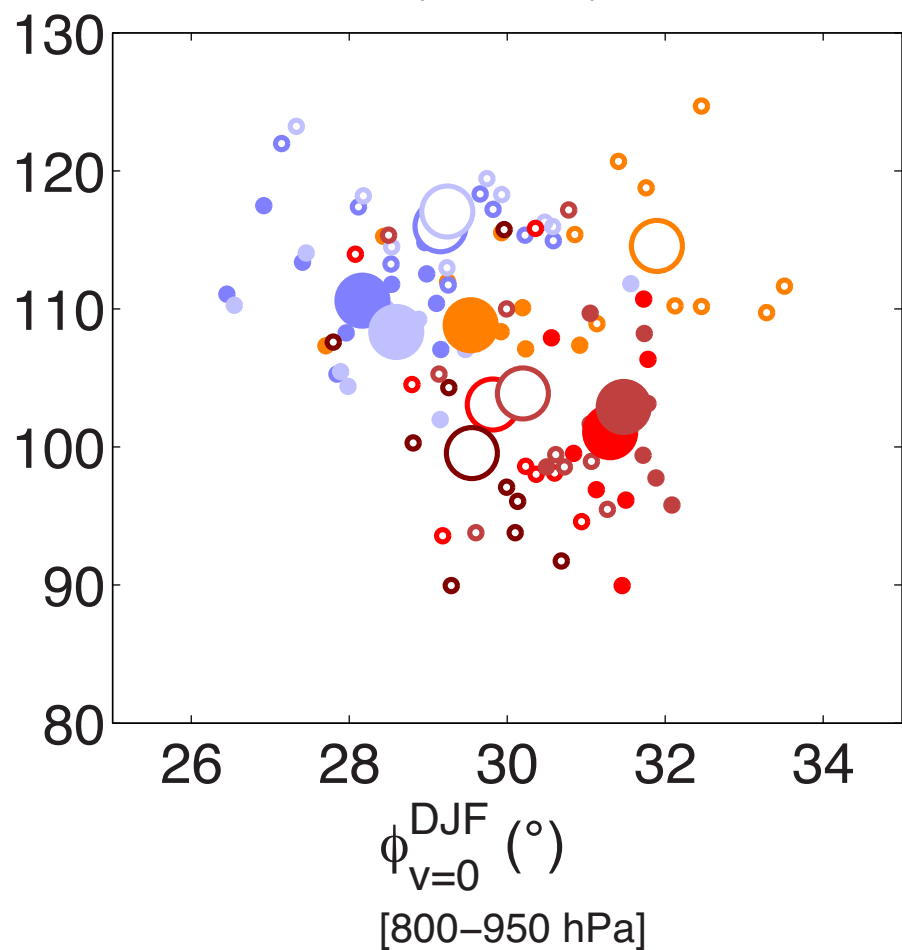
(d) DJF \phi_{v=0} - \chi_{\text{CO}} ( r = -0.26 )
