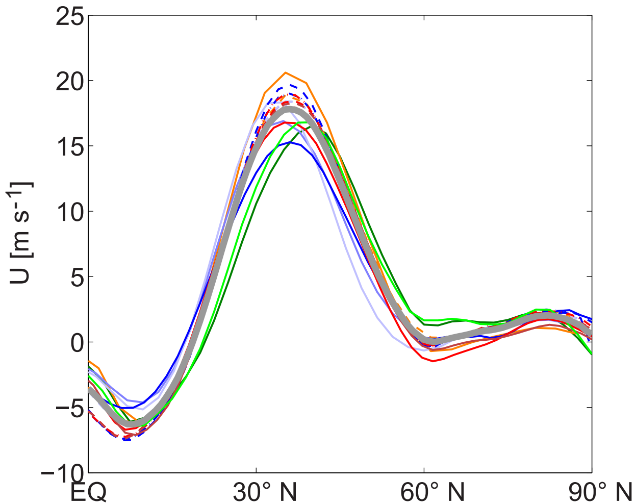
(a) DJF
