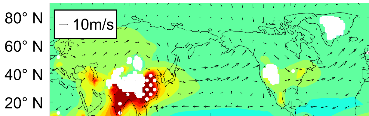
(a) 850 hPa, DJF
