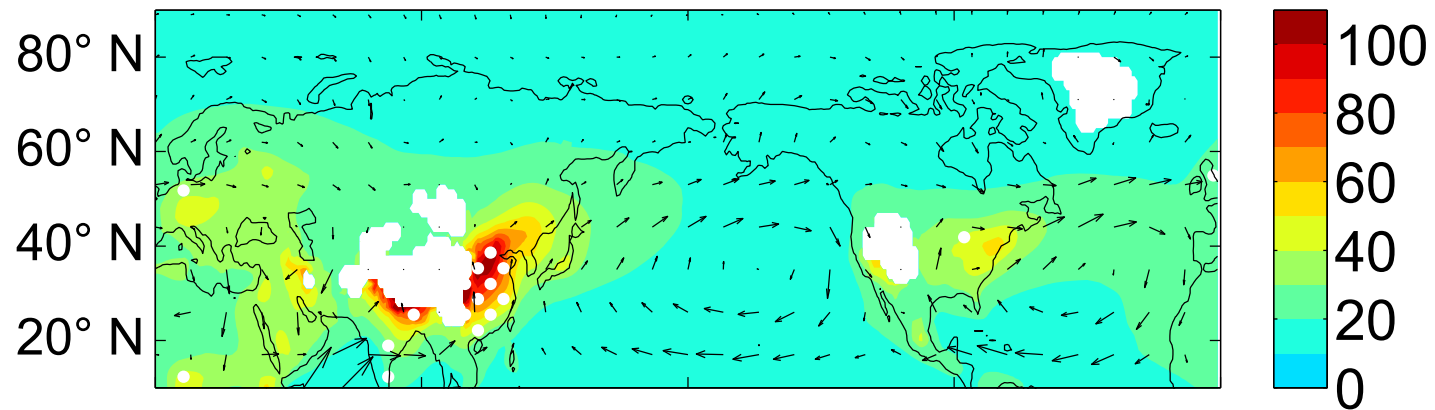
(d) 500 hPa, JJA
