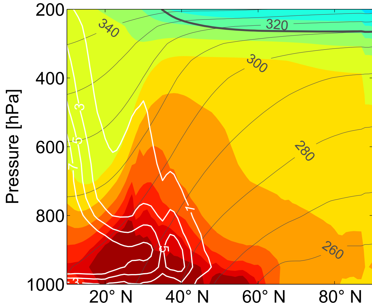
(e) DJF
