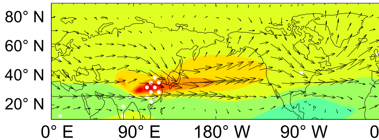
(e) DJF
