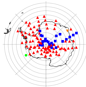
(d) CLaMS: 2011-06-25
