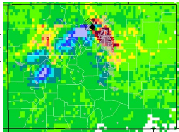
(d) Ethene
