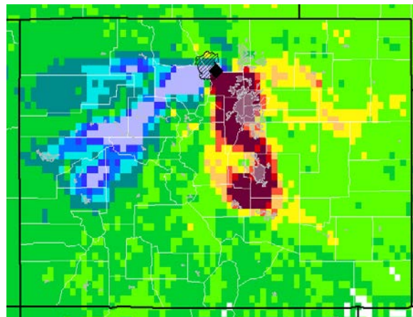
(b) C 2 Cl 4
