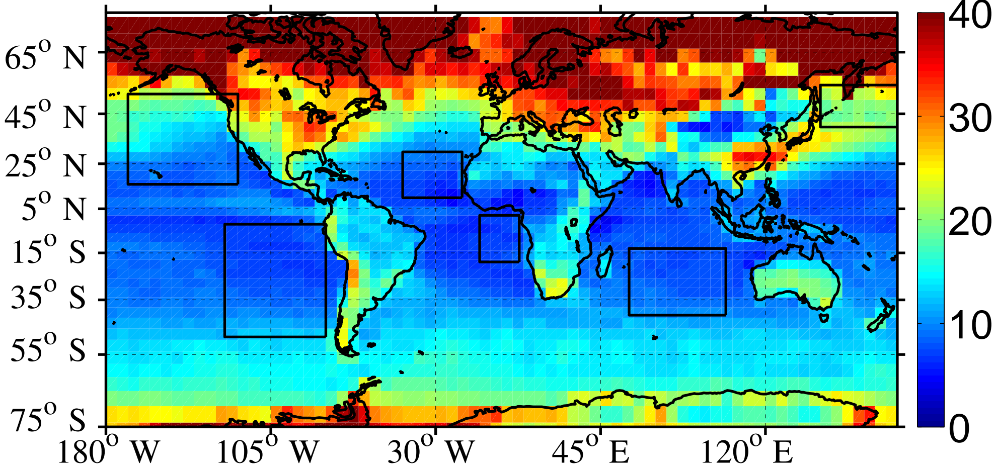
MODIS COD DJF
