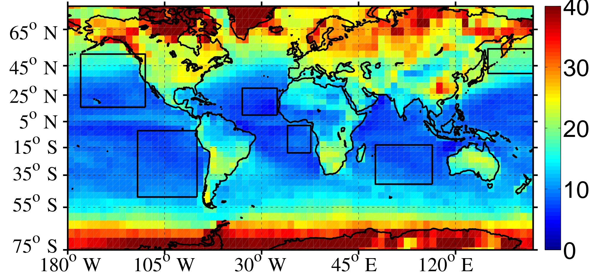
MODIS COD SON
