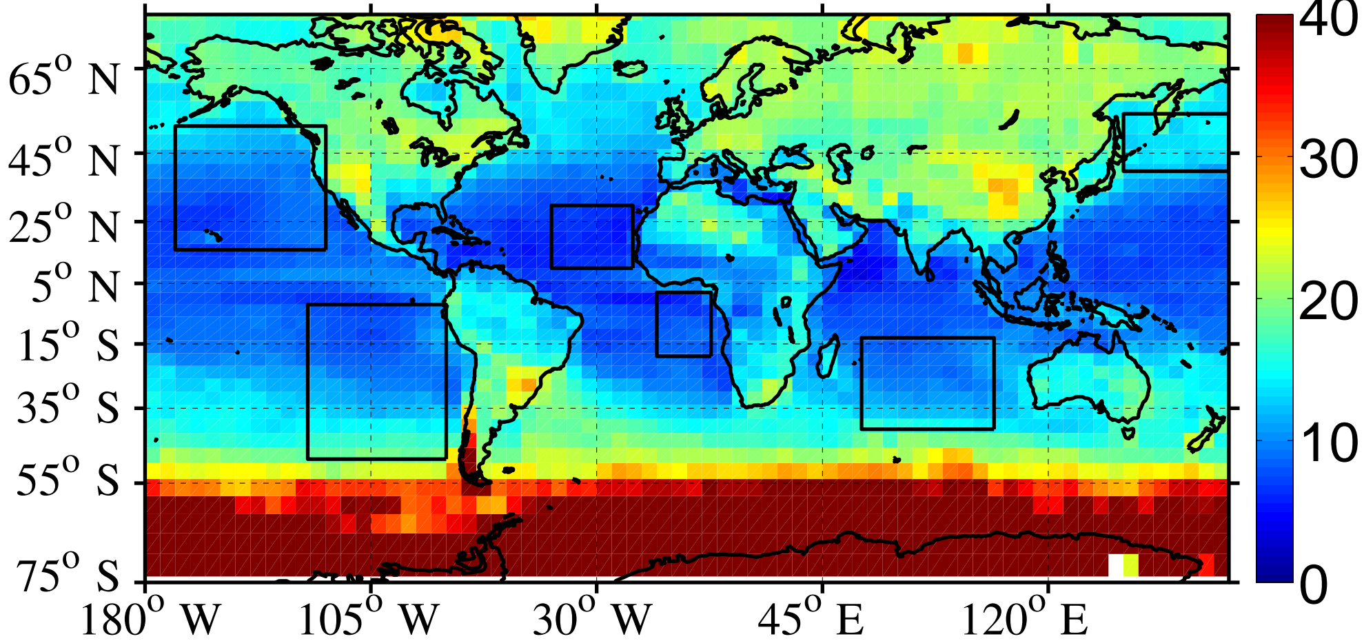
MODIS COD JJA
