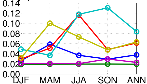
(d) CALIOP f_{AAC} \times \tau_{AAC}^{DR} (n. u.)
