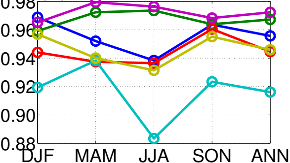
(e) Auxiliary SSA (n. u.)
