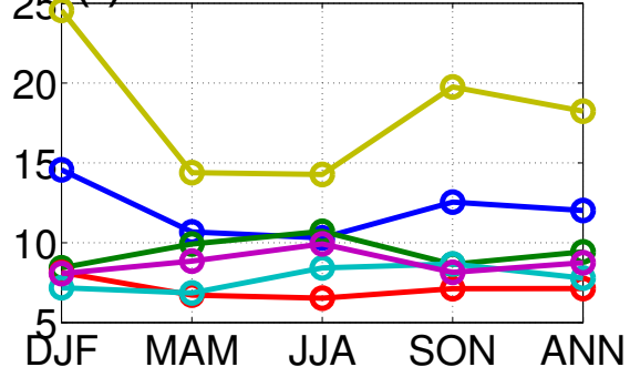
(f) Auxiliary COD (n. u.)
