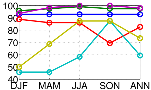
(d) CALIOP f_{AAC} \times \tau_{AAC}^{DR} (n. u.)
