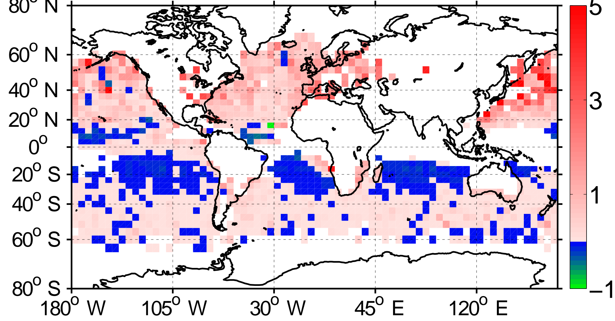
MAM min: -0.90 max: 5.72 mean: 0.20
