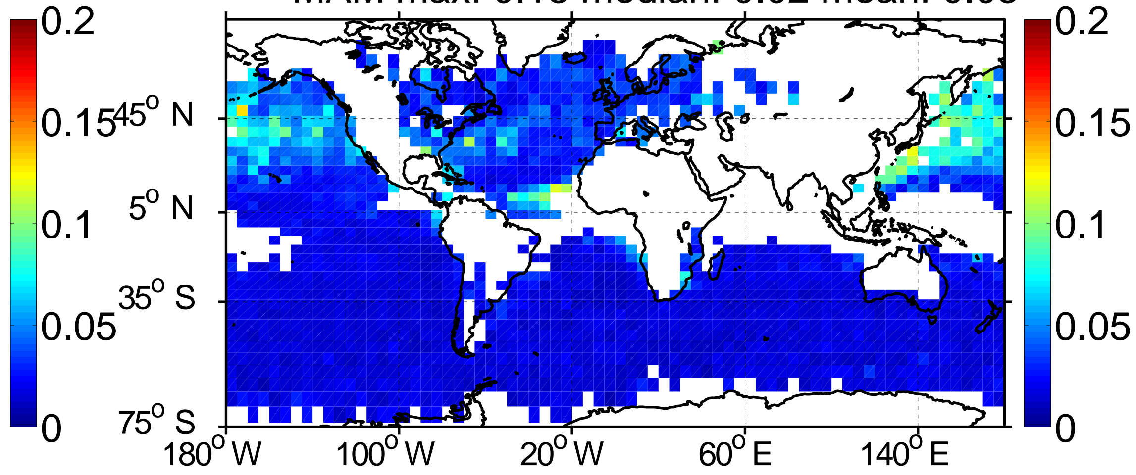
MAM max: 0.13 median: 0.02 mean: 0.03
