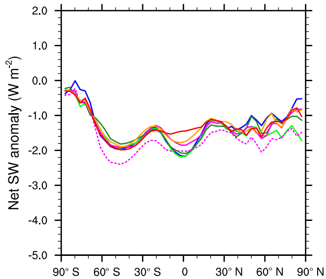
(d) Clear-sky SW forcing (SO 2 emission)
