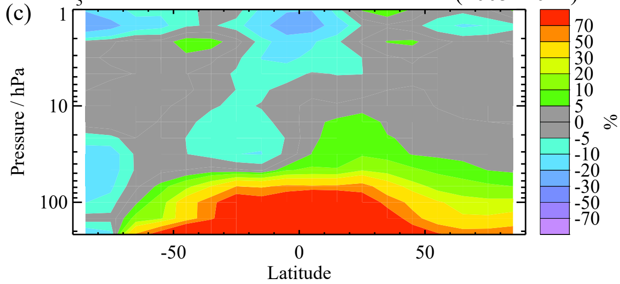
HNO 3 % Dif.: SD-WACCM - FR-WACCM (2005–2014)
