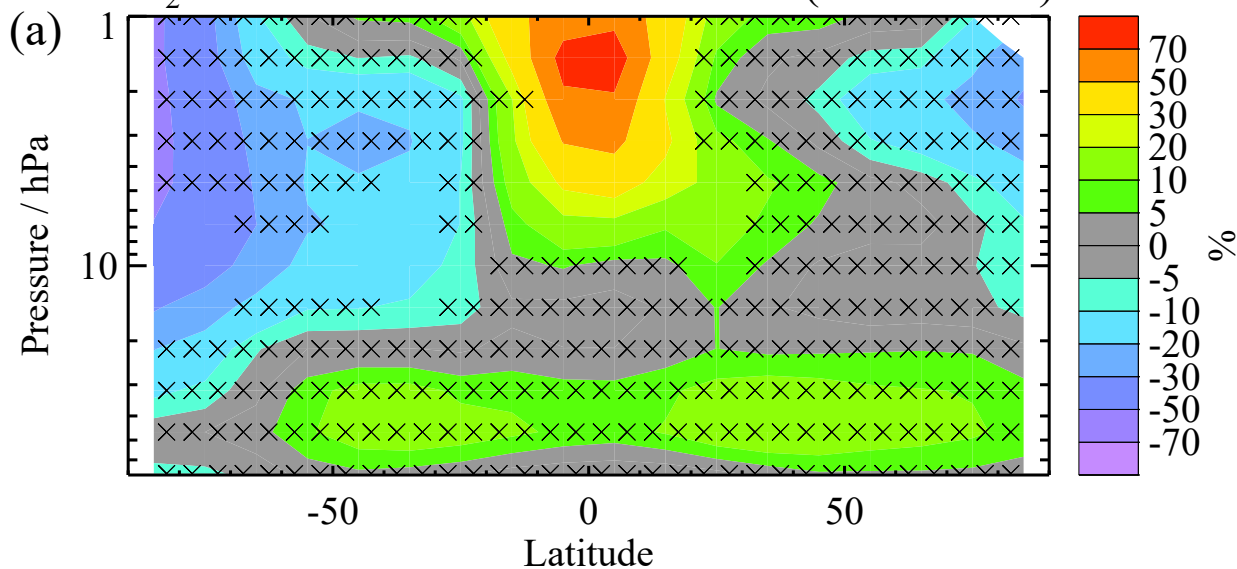
\text{N}_2\text{O} % Dif.: SD-WACCM - MLS (2005–2014)
