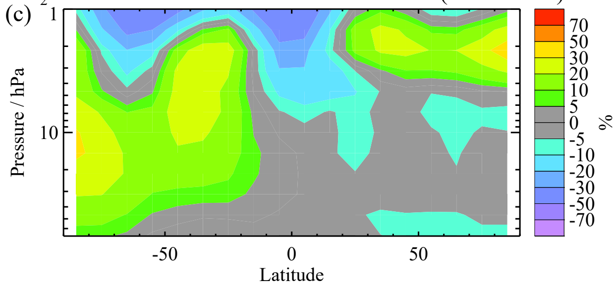
\text{N}_2\text{O} % Dif.: SD-WACCM - FR-WACCM (2005–2014)
