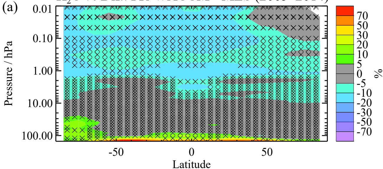
H 2 O % Dif.: SD-WACCM - MLS (2005–2014)
