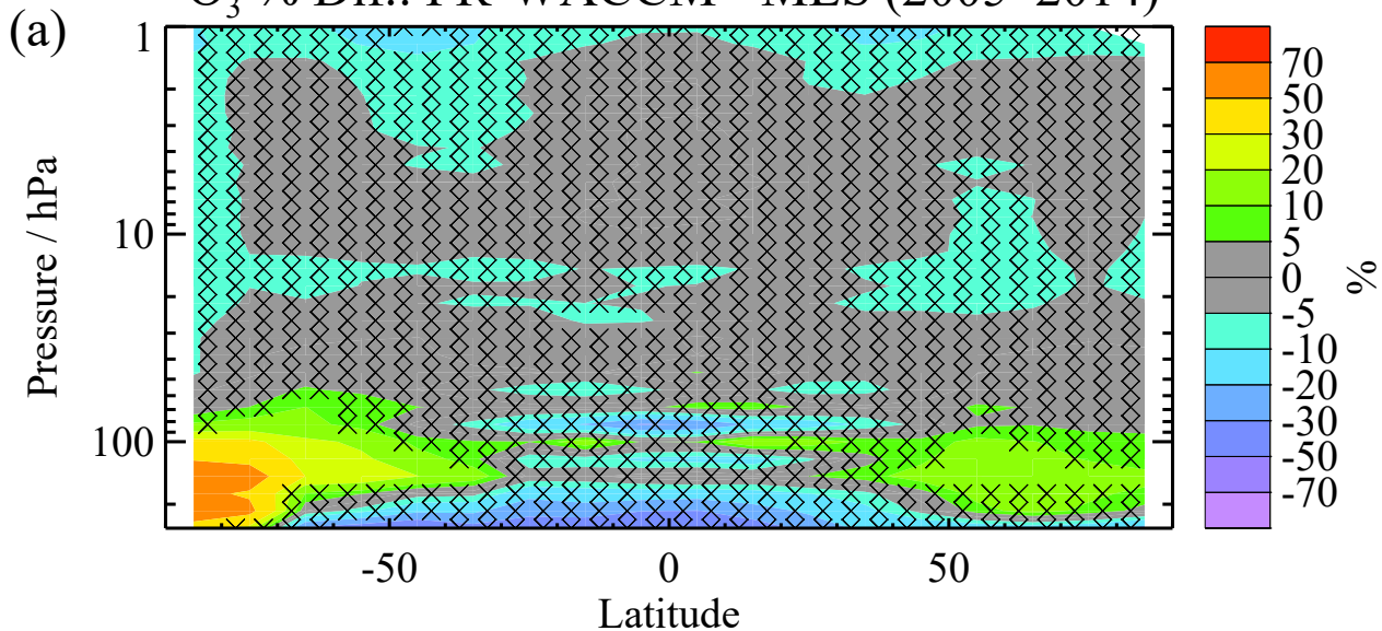
O 3 % Dif.: SD-WACCM - MLS (2005–2014)
