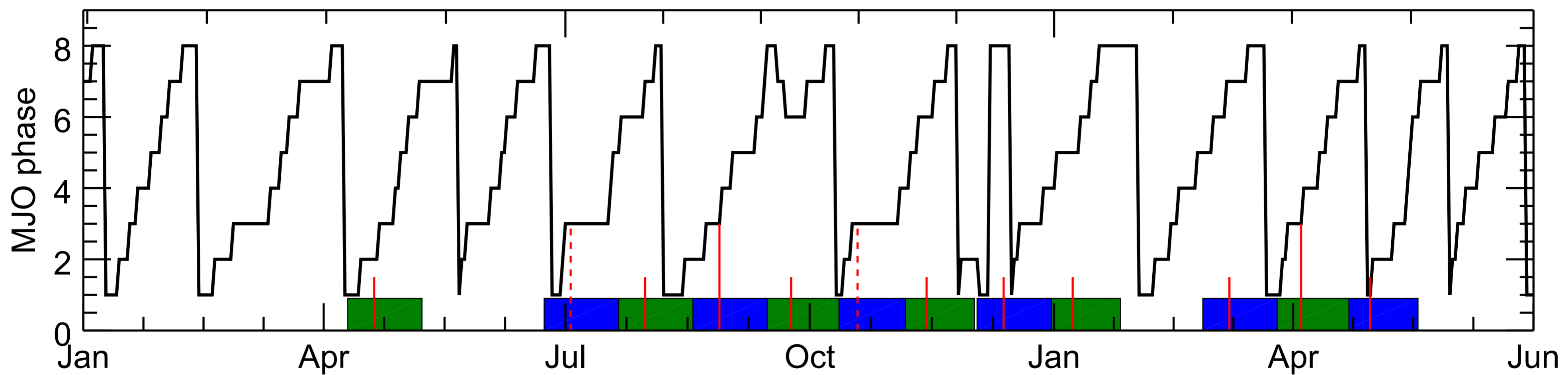
(b) MJO phase
