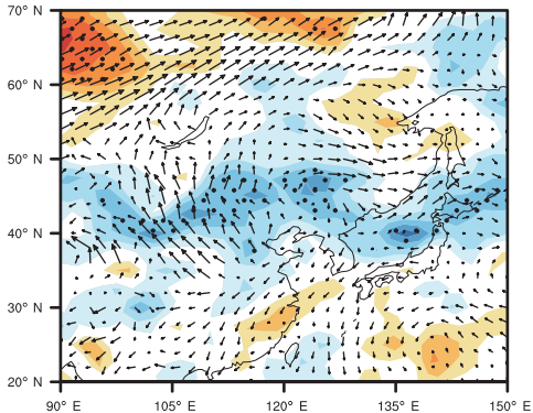
(d) Precipitation & wind sfc
