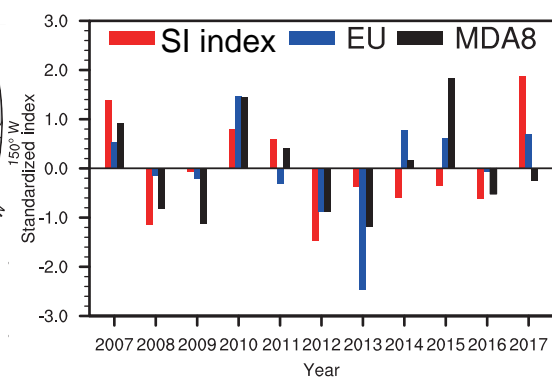
(b) SI index & EU & MDA8
