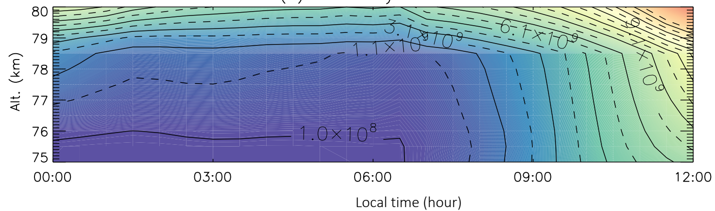
(d) O density \text{cm}^{-3}
