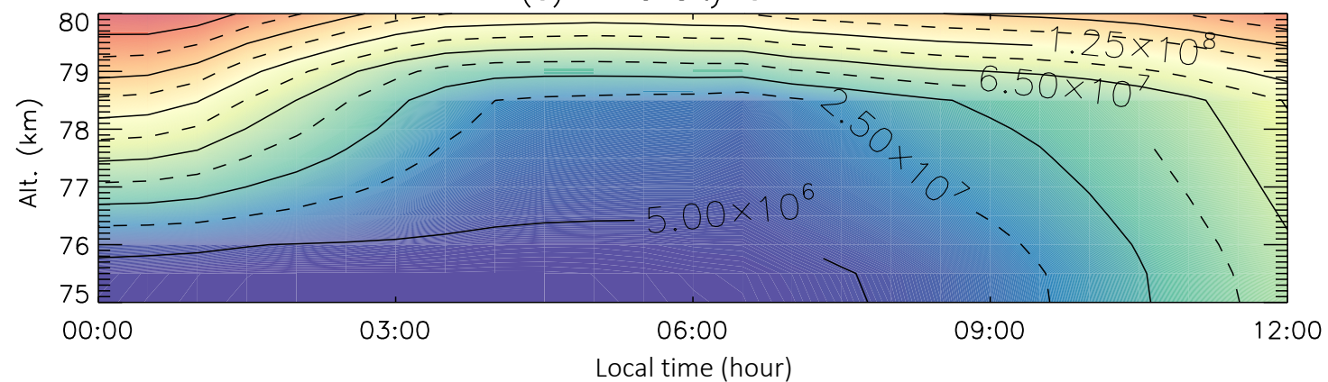
(d) O density \text{cm}^{-3}
