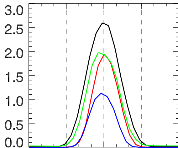
j(\text{O}^1\text{D}) / 10^{-5} \text{s}^{-1}
