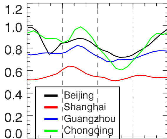
CO / ppmv
