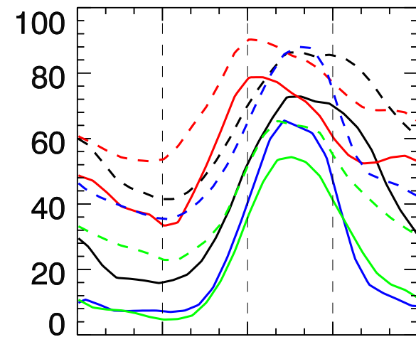
O 3 / ppbv
