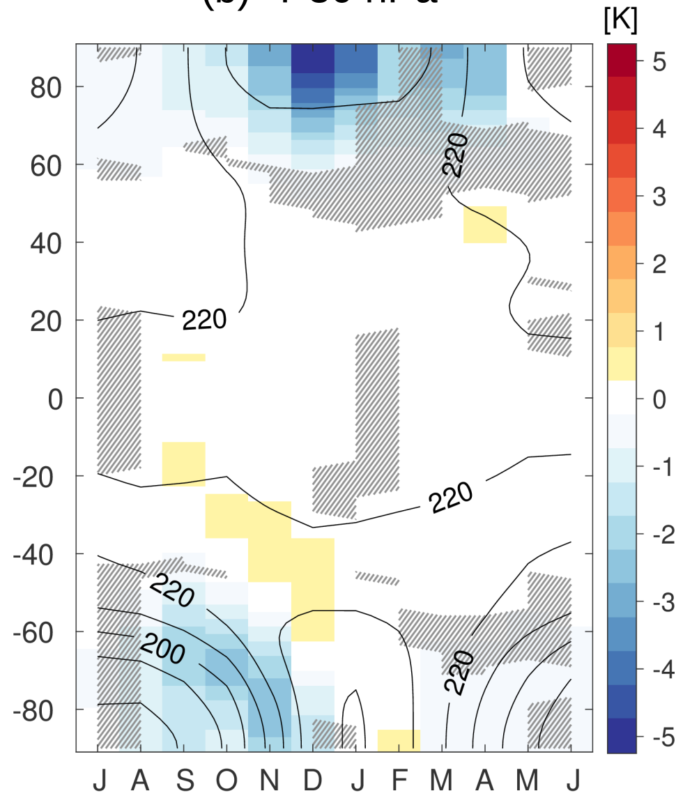
(b) T 30 hPa
