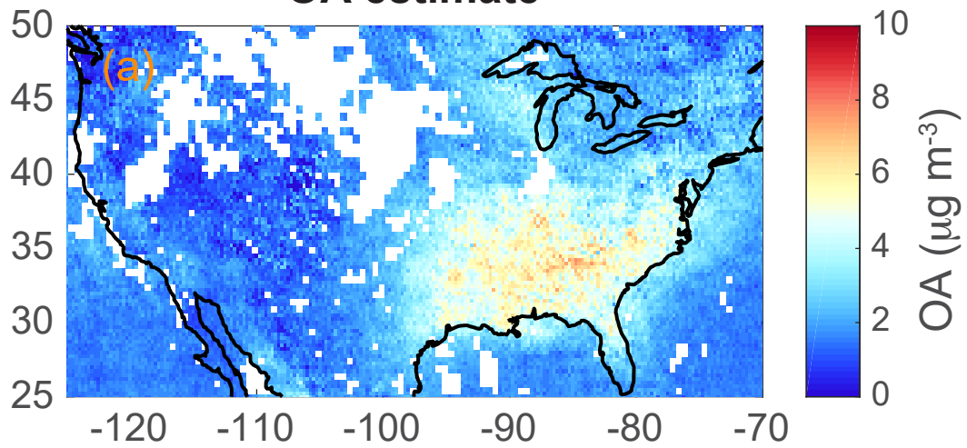
OA estimate
