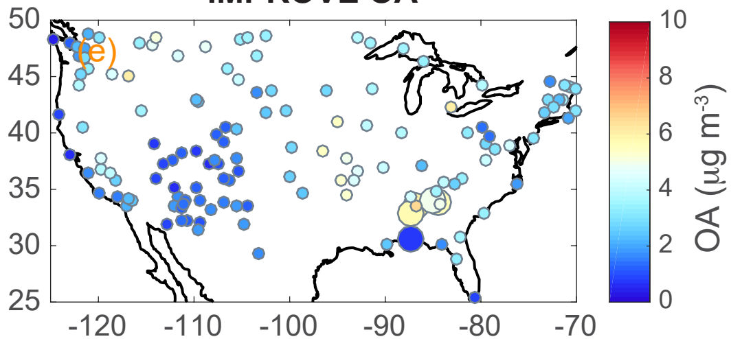
IMPROVE OA
