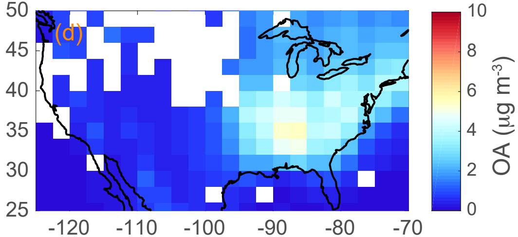
GEOS-Chem OA
